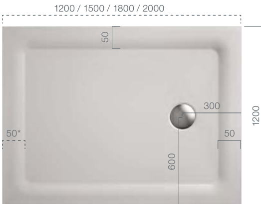
Bodengleich; *Funktionsrand (flexibel kürzbar)
