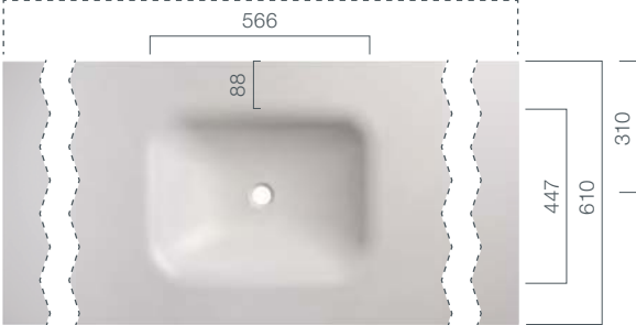
Becken mittig; Beckentiefe: 120 mm
