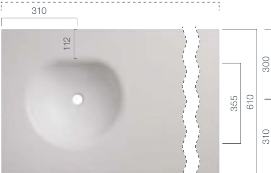
Becken links; Beckentiefe: 130 mm
