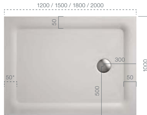
Bodengleich; *Funktionsrand (flexibel kürzbar)
