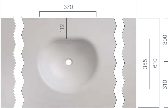
Becken mittig; Beckentiefe: 130 mm
