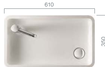
Beckentiefe: 60 mm; Gesamthöhe: 120 mm; Ø Armaturensockel: 50 mm
