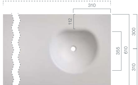
Becken rechts; Beckentiefe: 130 mm
