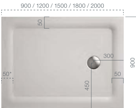
Bodengleich; *Funktionsrand (flexibel kürzbar)
